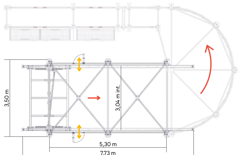
Montage anti-horaire
