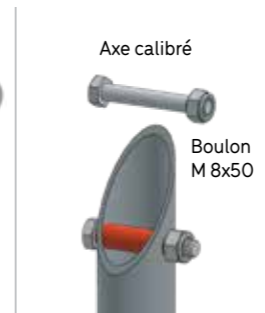
Bague inox anti-usure à l'articulation
