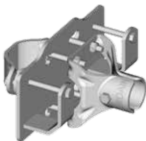
Bride TRÈFLE Ø 102 mm support raccordement écran frontal Ø 76 mm LO9924
